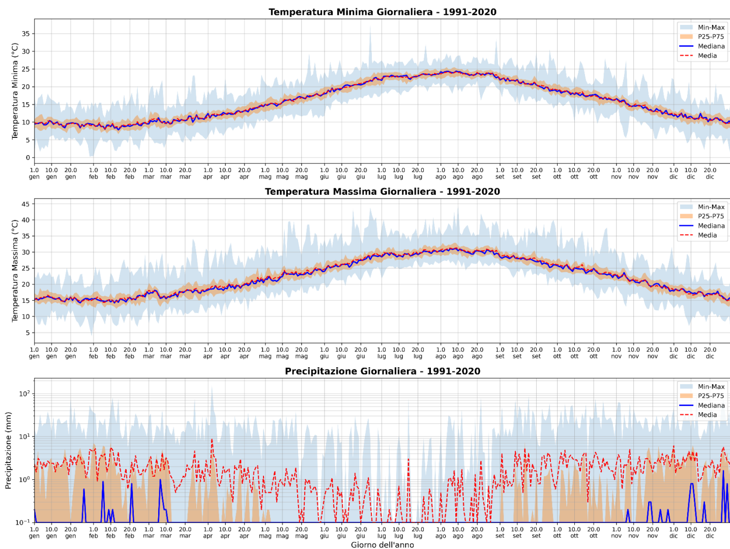
Figura 10: come in Figura 9, ma i dati sono riferiti al trentennio di riferimento 1991-2020.
