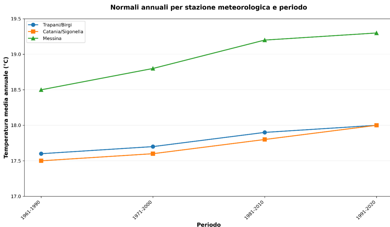
Figura 8: Normali annuali della temperatura media per tre stazioni siciliane (fonte ISPRA, vedi testo)
