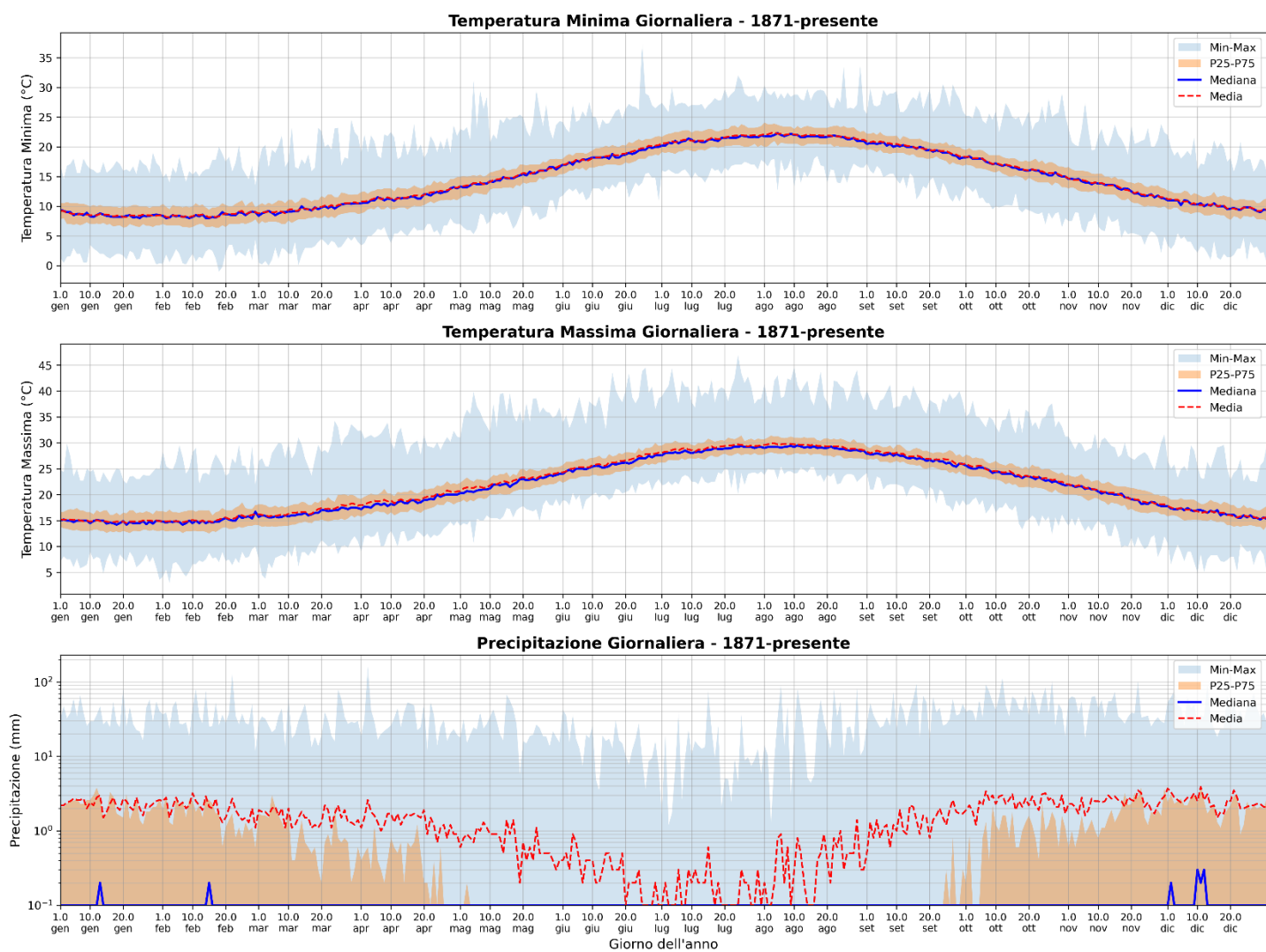
Figura 9: Valori giornalieri della temperatura massima, minima e delle precipitazioni derivate dall'analisi della serie di dati dal 1871 fino all'ultimo dato disponibile (Settembre 2025). Ogni figura mostra: l'intervallo minimo-massimo assoluto (area più chiara), l'intervallo interquartile P25-P75 (area più scura), la mediana (linea continua blu), la media (linea tratteggiata rossa). L'ordinata del grafico relativo alle precipitazioni è in scala logaritmica per mostrare l'ampio range dinamico fra i minimi ed i massimi. Al solo fine della rappresentazione, in questo grafico valori \leq 0.1 mm sono considerati tutti pari a 0.1.
