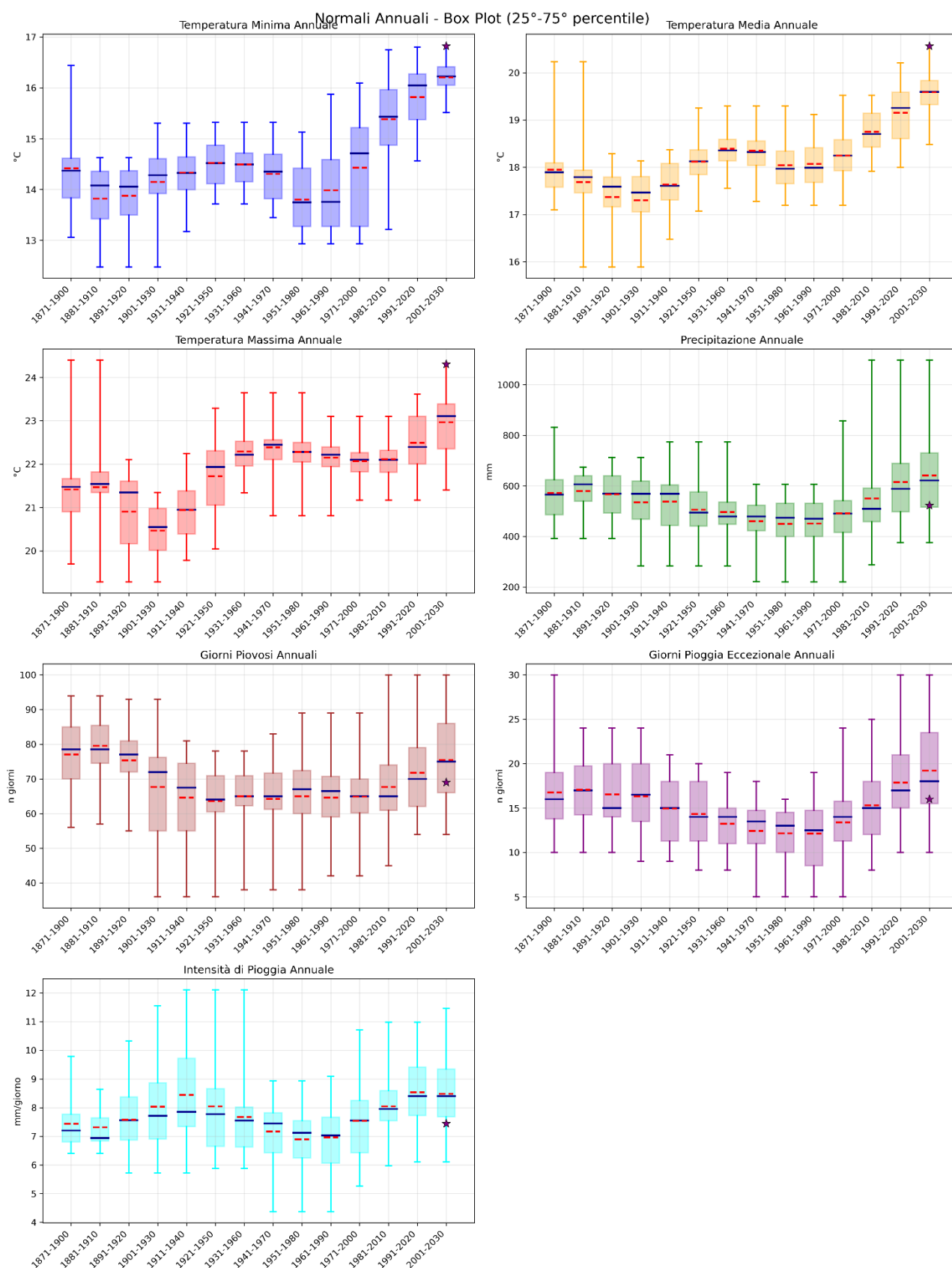
Figura 8: Normali annuali di tutte le quantità riportate nelle figure precedenti. Le box rappresentano il 25° ed il 75° percentile ed i whiskers il valore massimo delle medie annuali degli anni del rispettivo trentennio. La stella rappresenta i valori del solo anno 2024.
